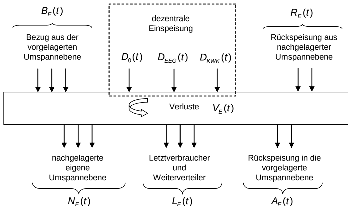
Bild 1-1: Netzmodell zur Herleitung der vermiedenen Netzentgelte einer Netzebene
